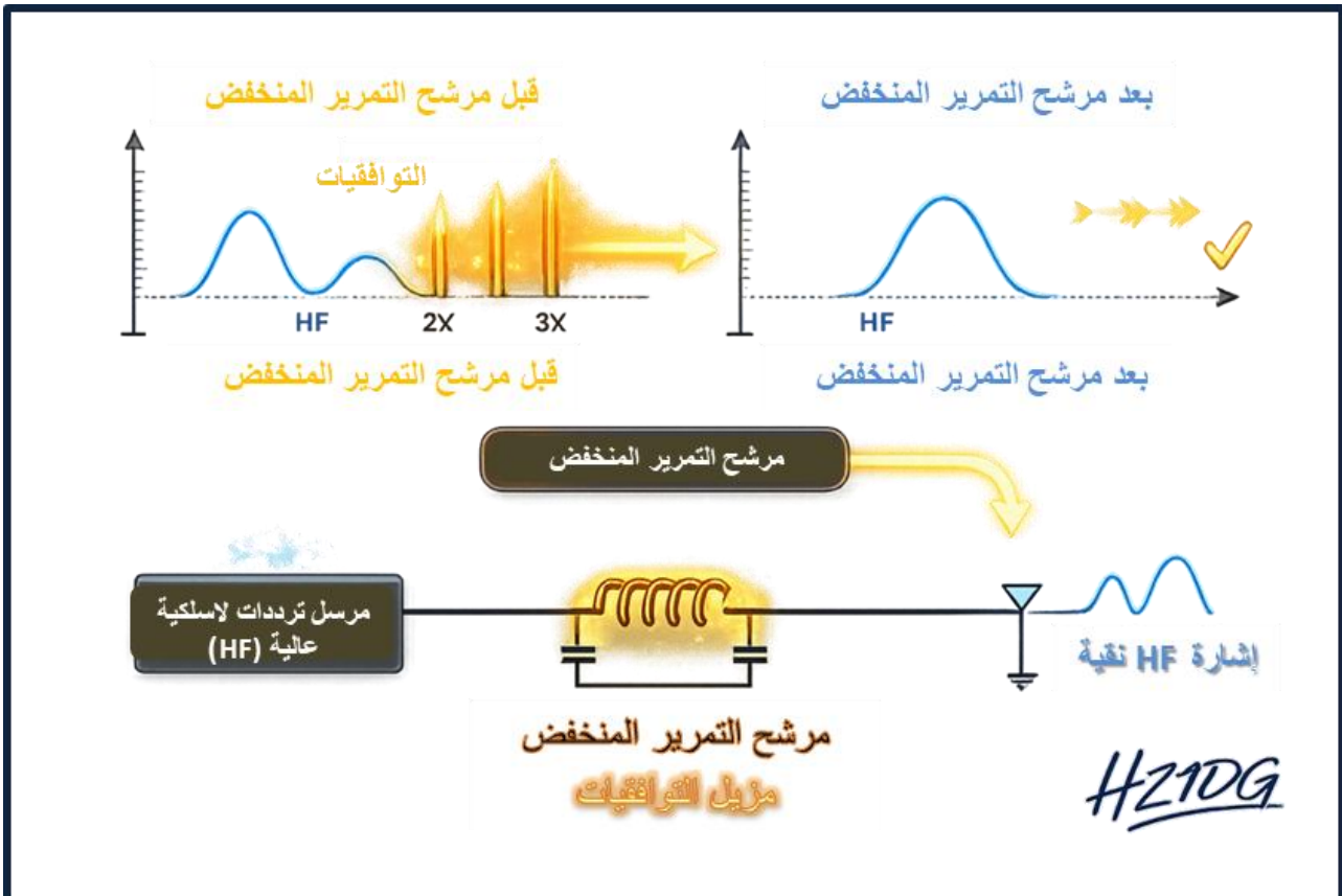
شكل (10-6): تأثير المرشح منخفض التمرير (Low-Pass Filter) على الإشارة وإزالة التوافقيات
