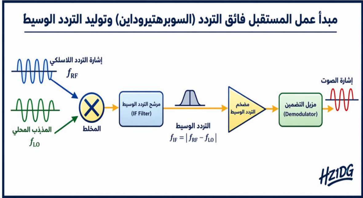
شكل (2-7): مبدأ المزج في مستقبل Superheterodyne وتوليد (IF).
