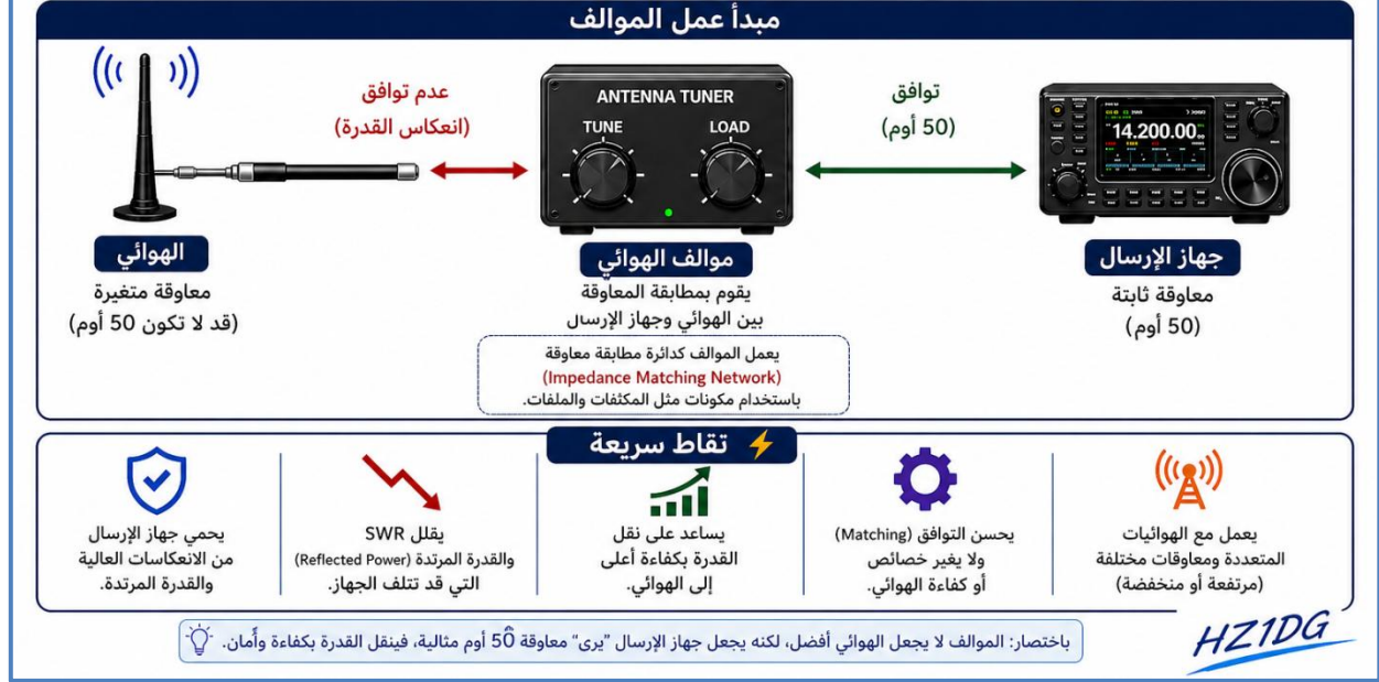
شكل (3-8): مبدأ عمل الموالف
