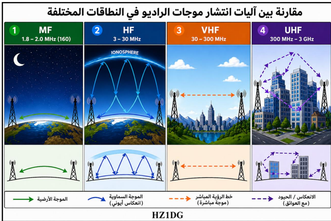
شكل (2-2) : مقارنة بين آليات انتشار موجات VHF و HF و UHF .
