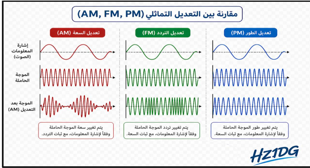
شكل (5-7): مقارنة بين AM و FM و PM
