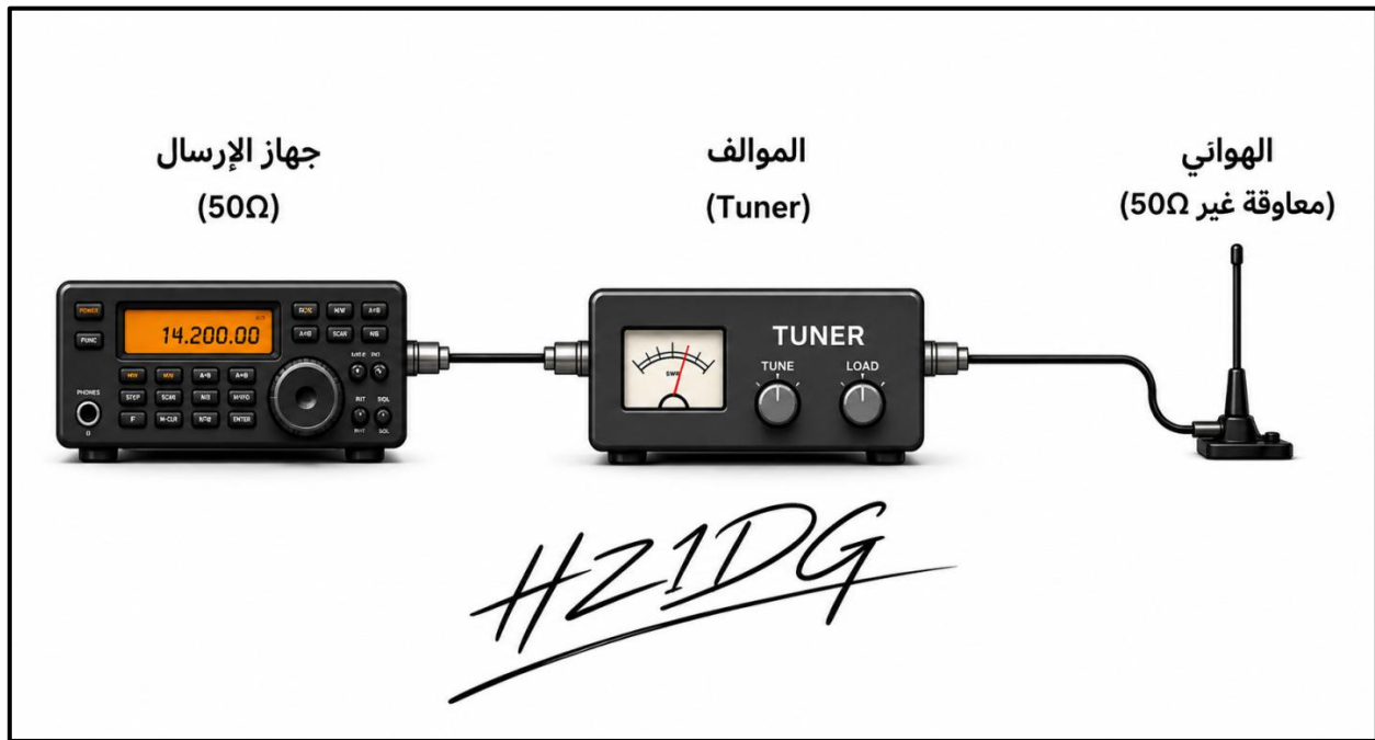
شكل (2-8): استخدام الموالف لمطابقة المعاوقة بين جهاز الإرسال (50 أوم) وهوائي غير متوافق.
