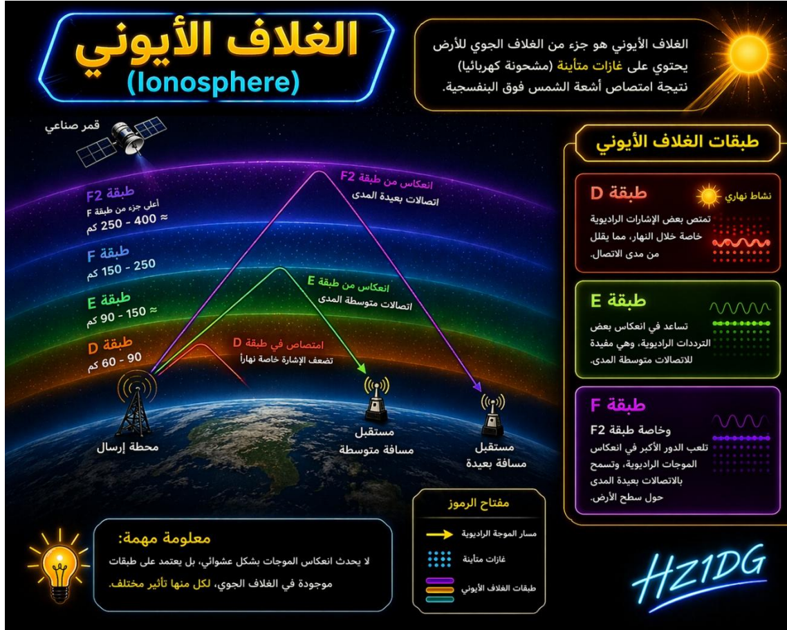
شكل (2-5): طبقات الغلاف الأيوني وتأثيرها على انتشار الموجات
