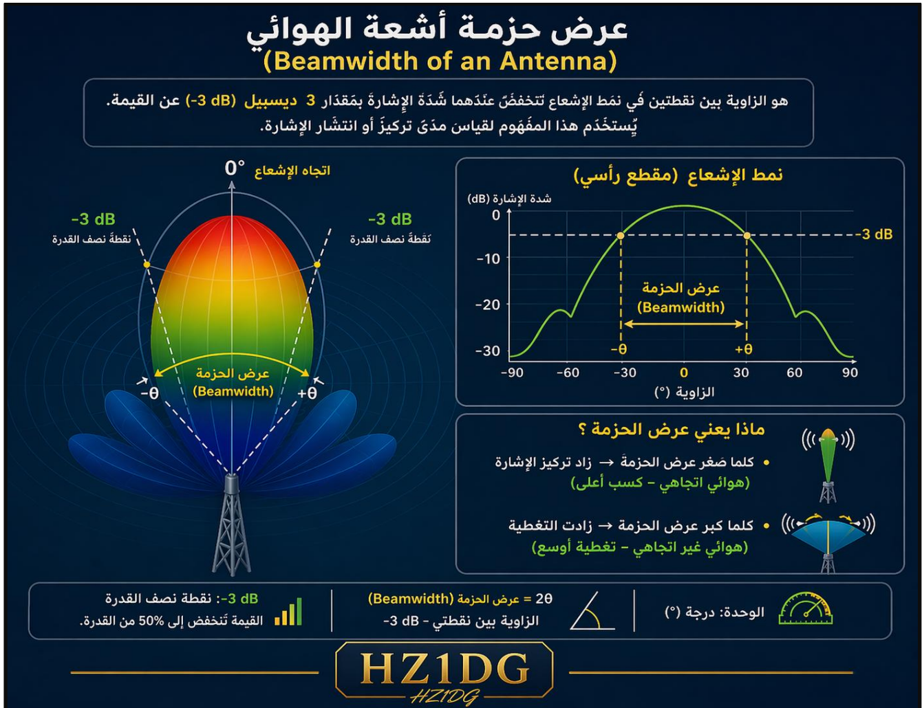
شكل (8-10): عرض حزمة أشعة الهوائي
