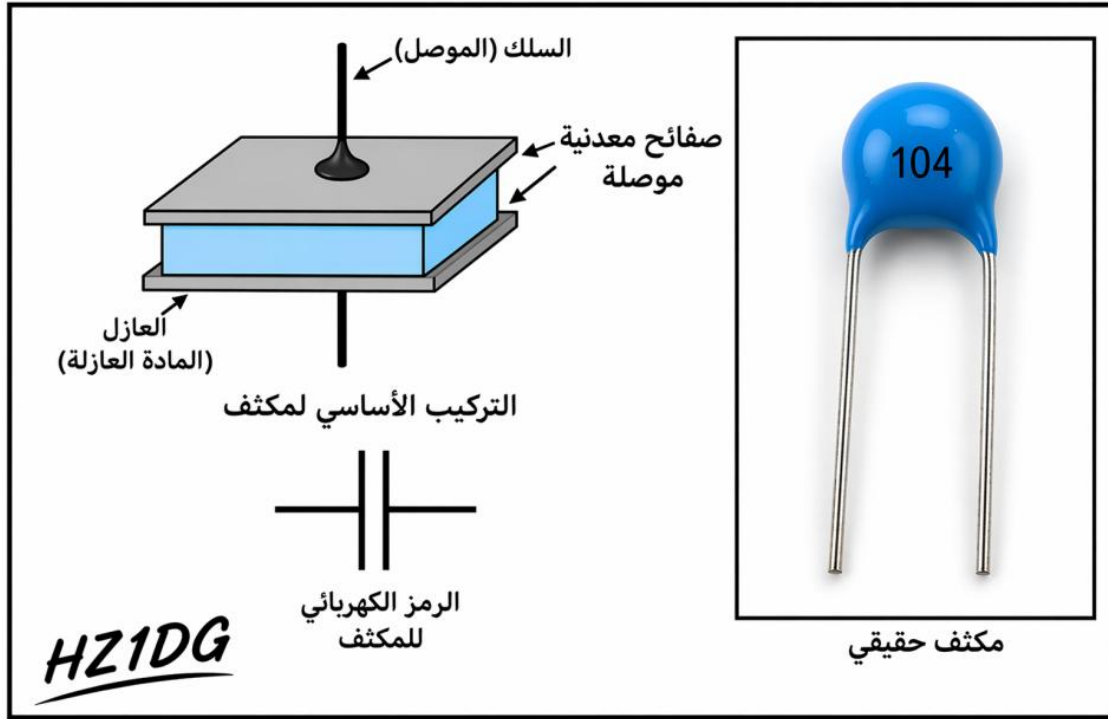
شكل (4-6): البنية الأساسية للمكثف وتمثيله الرمزي
