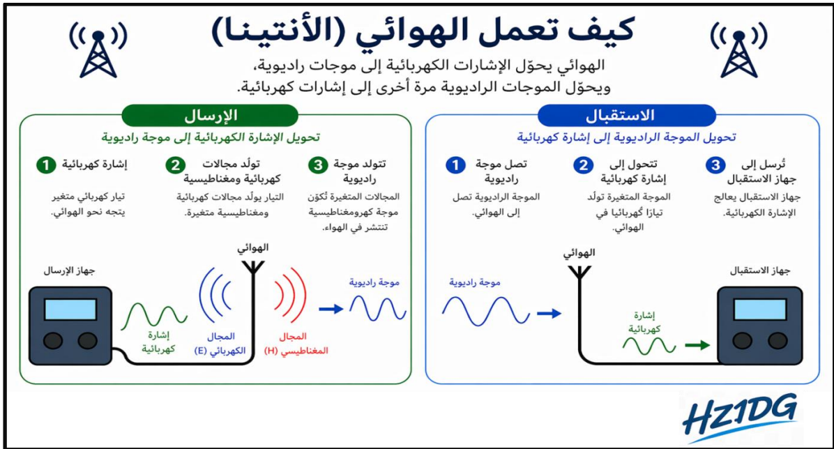
شكل (1-8): مبدأ عمل الهوائي
