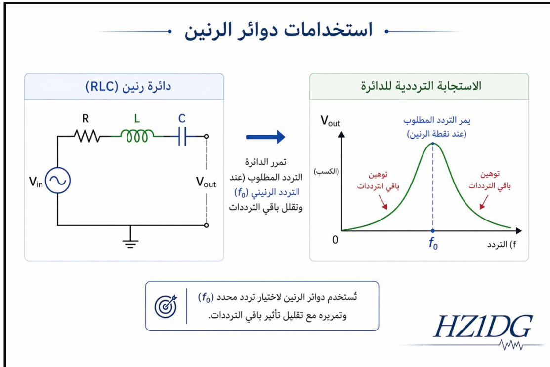
شكل (6-11): دوائر الرنين واستخدامها في تحديد التردد المطلوب
