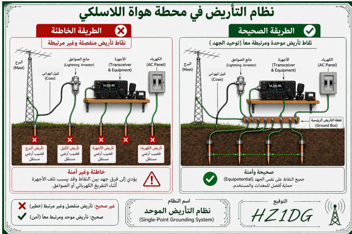
شكل (2-9): نظام التأريض لمحطة لاسلكي
