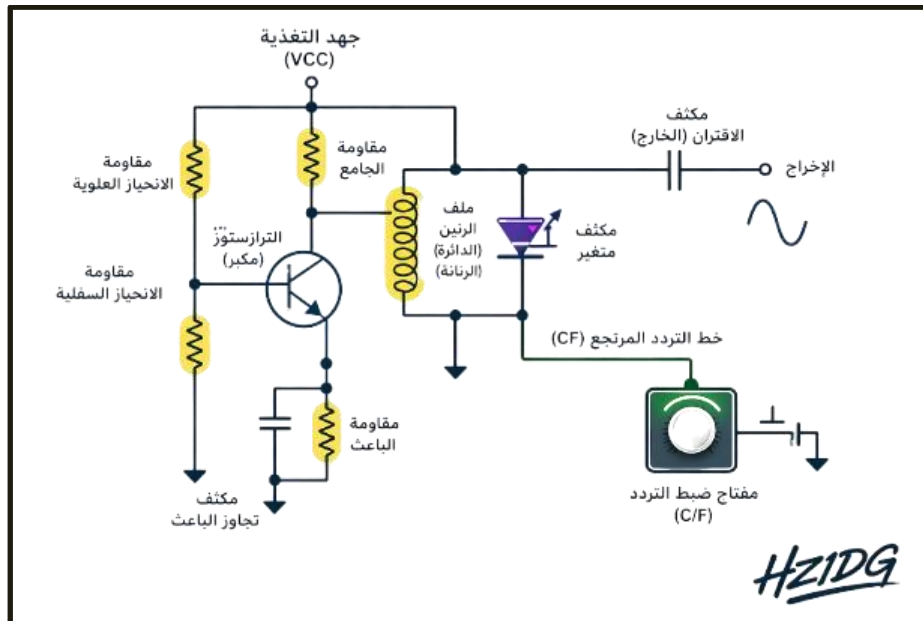
شكل (9-6): مذبذب متحكم بالجهد (VCO)
