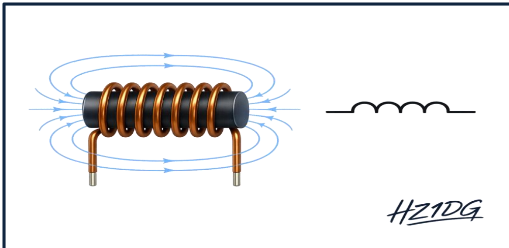
شكل (6-6): الملف (Inductor) والمجال المغناطيسي حوله ورمزه
