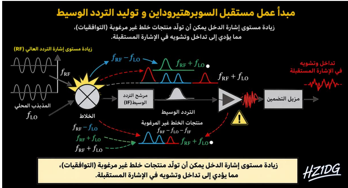
شكل (3-7) : تأثير النواتج التداخلية للمزج على جودة الاستقبال
