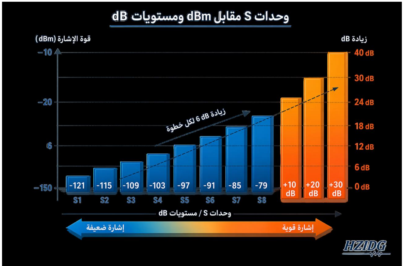
شكل (7-10): رسم بياني لمقياس الإشارة بعد S9 (S-Meter +dB)
