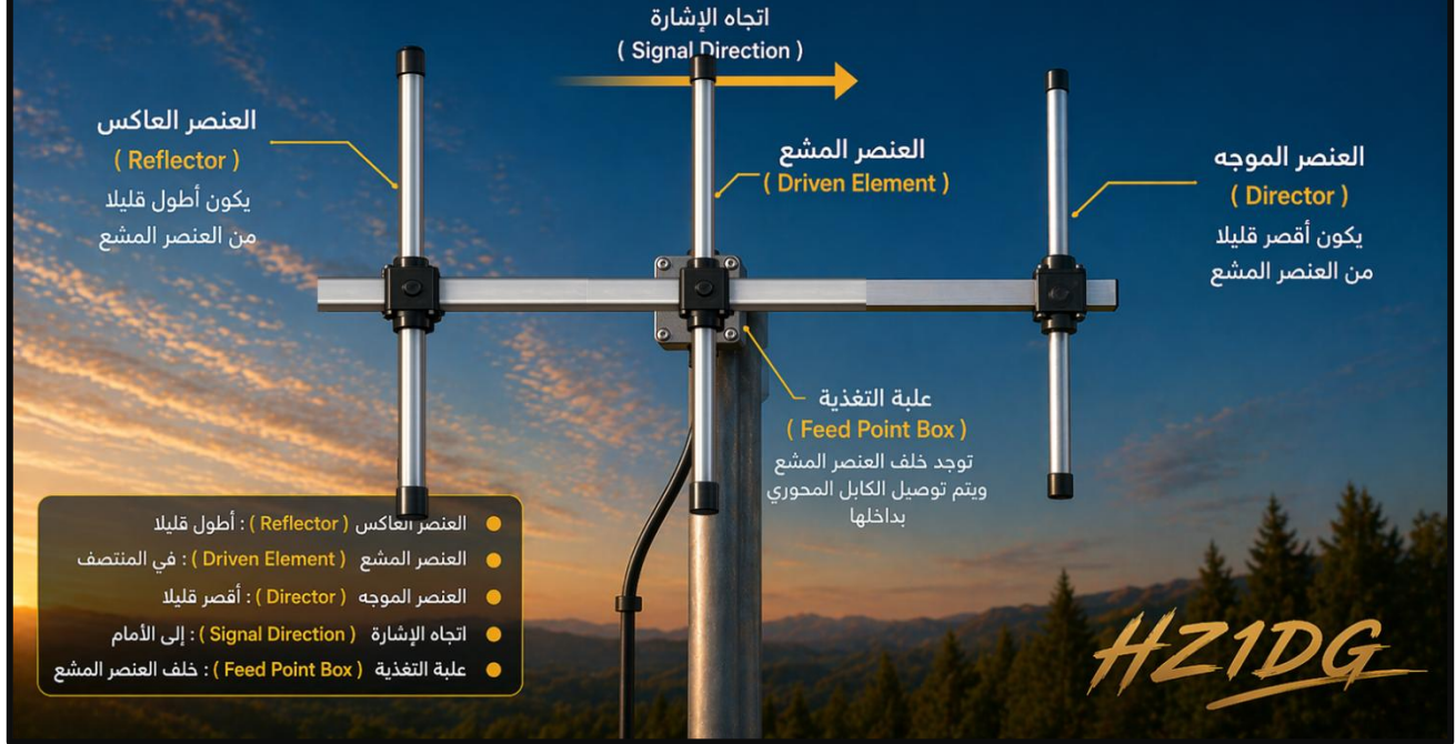
شكل (5-8): هوائي توجيهي - ياغي
