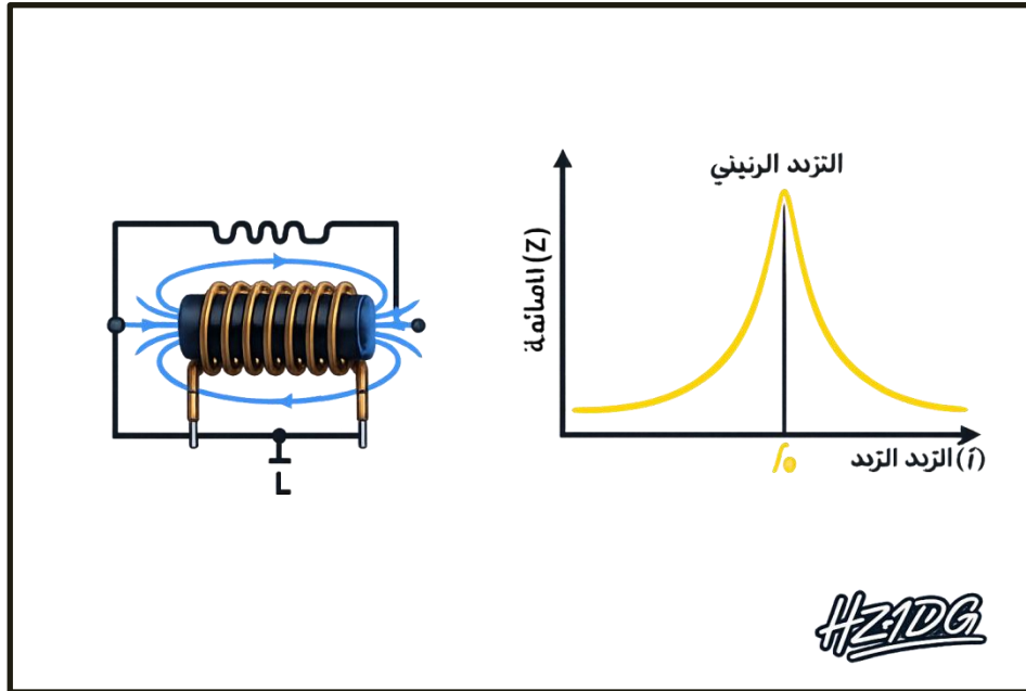
شكل (8-6): منحنى الرنين وعلاقته بالتردد
